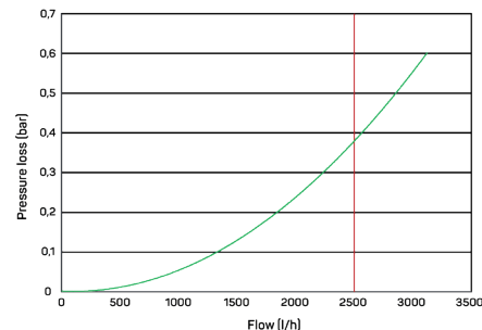
Curva tipica della perdita di pressione - DN15 R400
